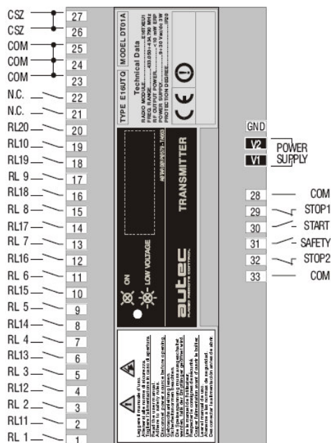
Sendereinheit
